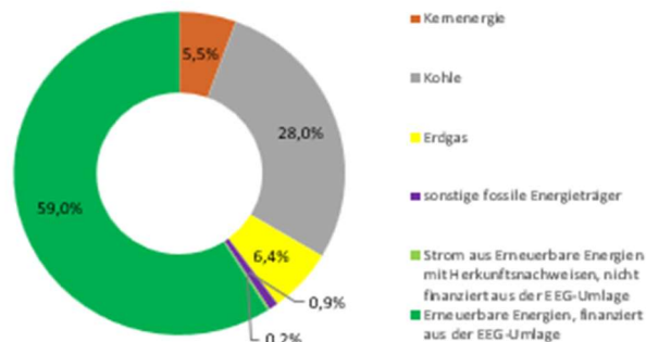
Verbleibender Energieträgermix DSDL alle sonstigen Produkte und Tarife 2022
